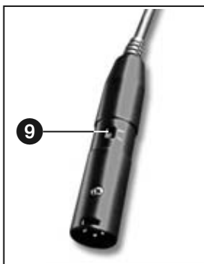
Abb. 1a: Phantomspeiseadapter mit Bassabschwächungsschalter (9)
