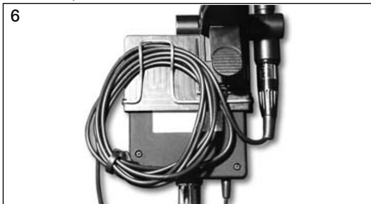
Fig. 4: Enrolar e fixar o cabo de conexão
